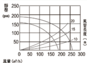
規格曲線
